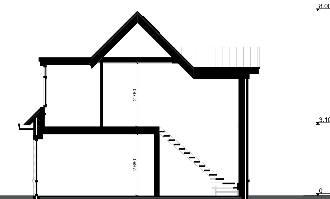
Principe doorsnede (1:100)
