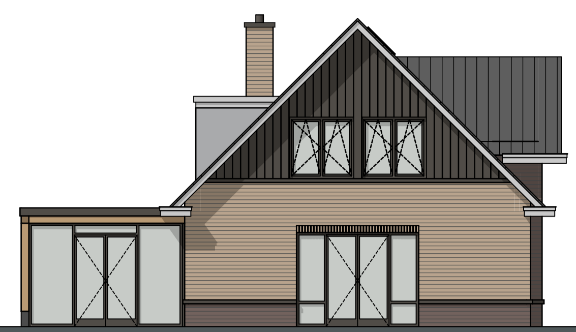
Voorgevel (1:100)
