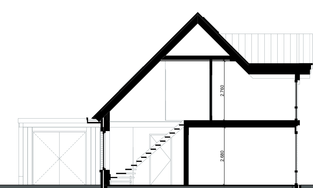
Principe doorsnede (1:100)
